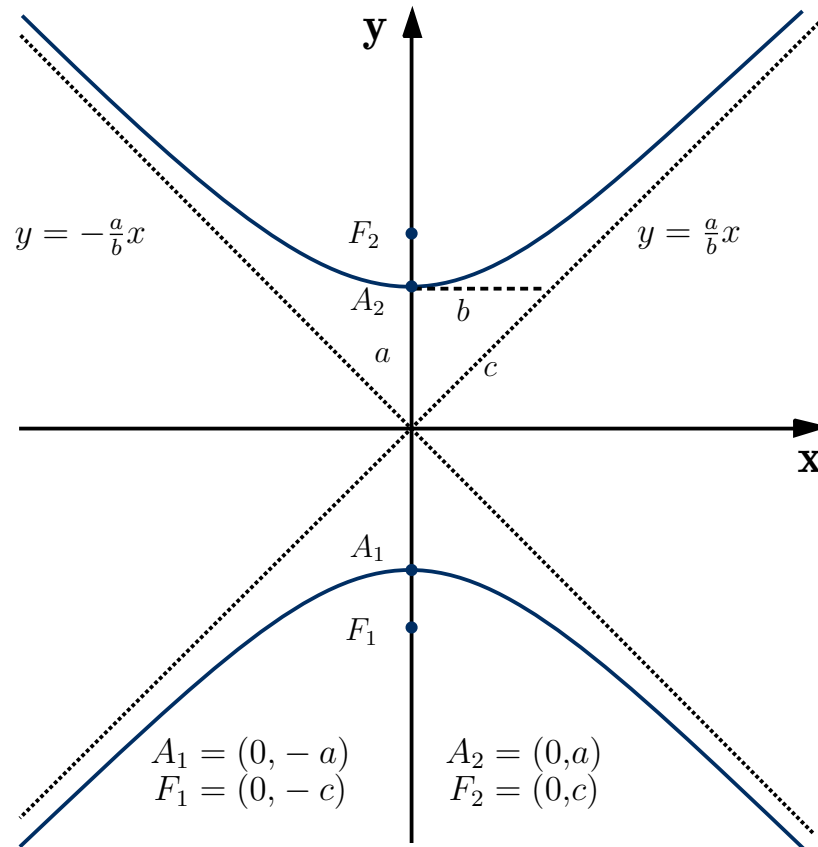
Figura 3.3: Hipérbole com focos F_1 = (0, -c) e F_2 = (0, c)
