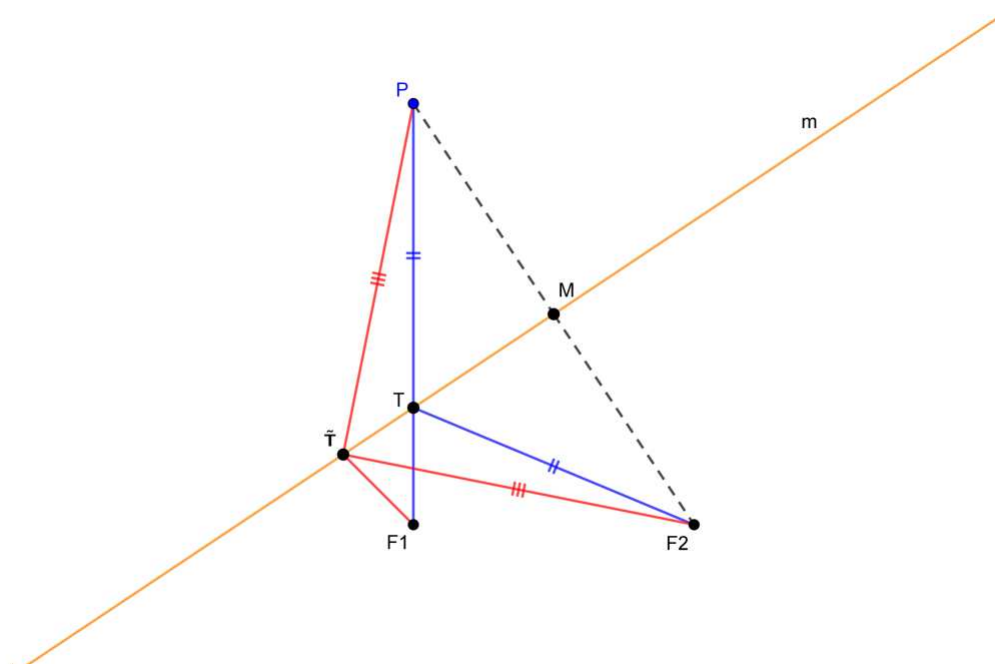
Figura 5.4: Representação da congruência dos triângulos \Delta\tilde{T}MF_2 e \Delta\tilde{T}MP
