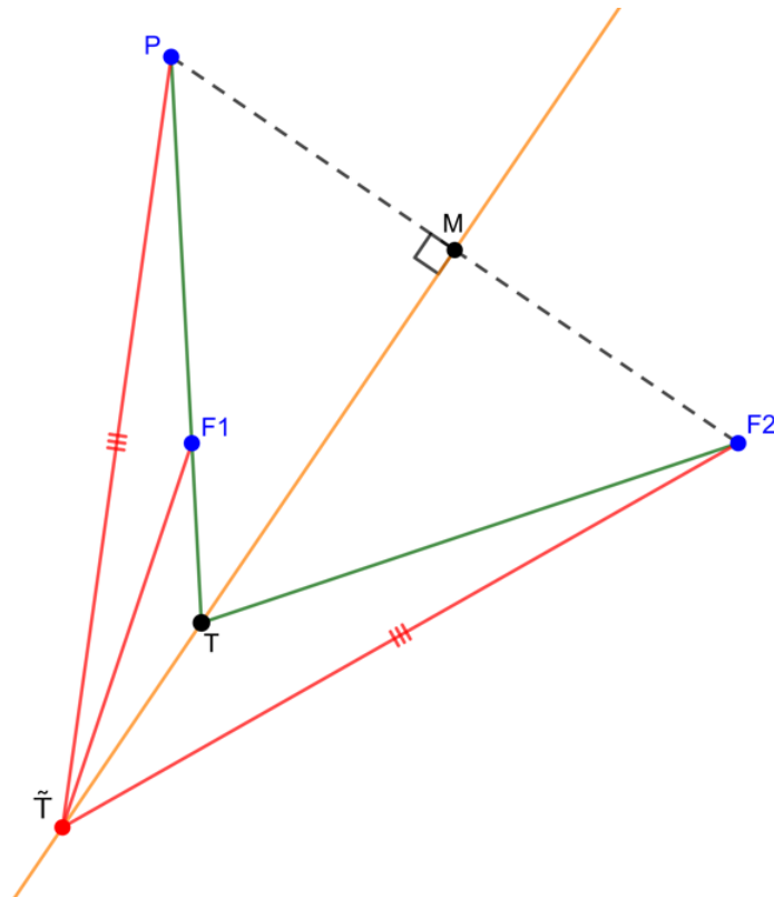
Figura 5.6: Representação da congruência dos triângulos \Delta\tilde{T}MP e \Delta\tilde{T}MF_2
