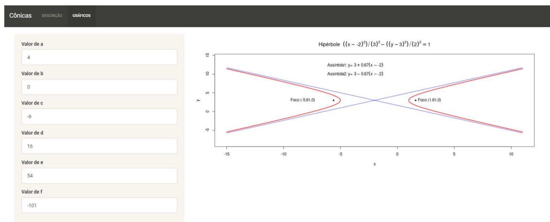
Figura 5.8: Gráfico da Hipérbole Gerada no Aplicativo a Partir da Escolha de Alguns Coeficientes da Equação Geral
