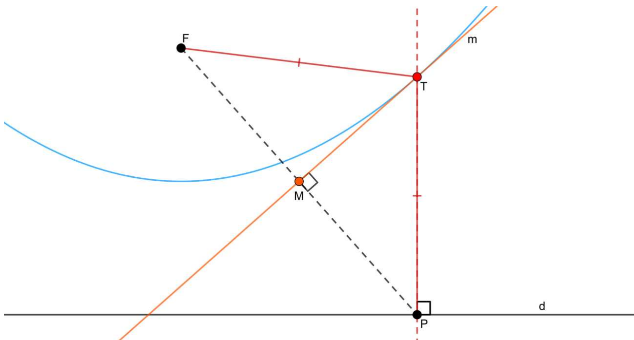
Figura 5.1: Mediatriz de P e F
