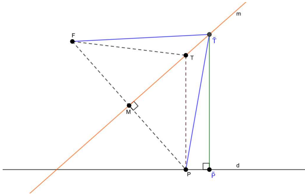
Figura 5.2: A projeção de \tilde{T} sobre d
