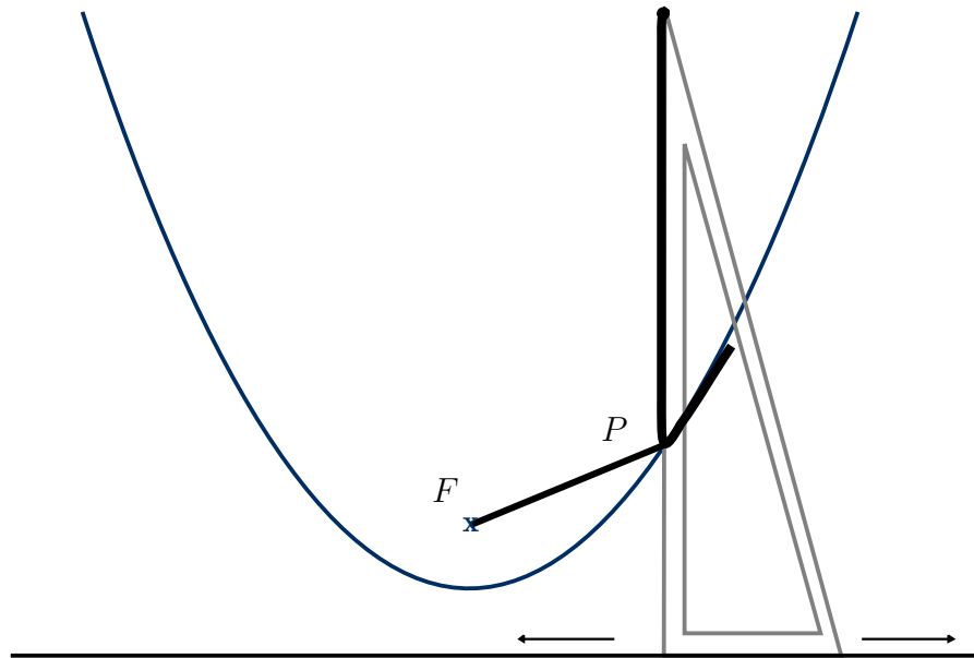
Figura 3.4: Conjunto dos pontos P = (x,y) tais que dist(P,F) = dist(P,r)
