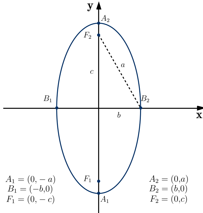
Figura 3.2: Elipse com foco nos pontos F_1 = (0, -c) e F_2 = (0,c)
