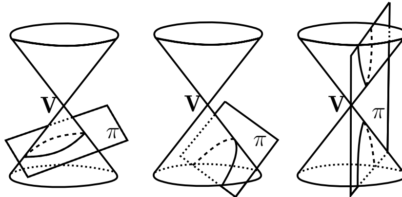
Figura 3.1: Secção Cônica que apresenta a Elipse, a Hipérbole e a Parábola. Base para a demonstração do Teorema de Dandelin
