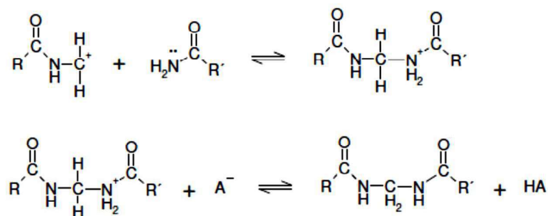
Figura 13. Formação de pontes metilênicas. Fonte: LESSMANN (2008).
