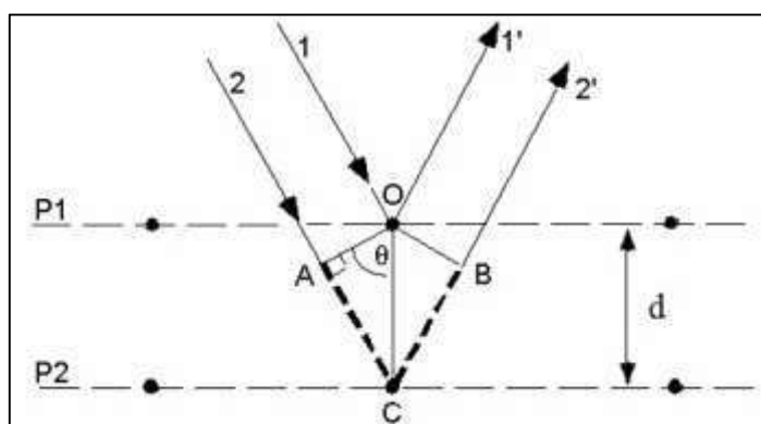
Figura 7. Fenômeno de difração de raios-X sobre um material cristalino. Fonte: Adaptado de MONTEIRO (2017).
