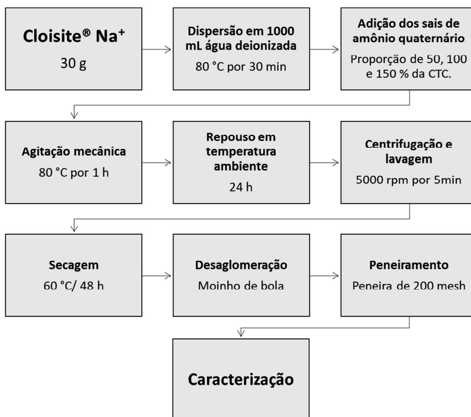
Figura 16. Fluxograma da modificação orgânica da nanoargila em dispersão aquosa.
