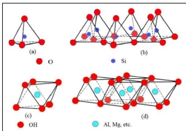
Figura 2. Representação de um tetraedro de silício [ \text{SiO}_4 ] (a), que forma uma folha tetraédrica (b) ao compartilhar os seus vértices com outros tetraedros, e de um octaedro [ \text{M}(\text{OH})_6 ] (c) que forma uma folha octaédrica (d) ao compartilhar as arestas com outros octaedros. Fonte: Adaptado de MANGONI et al. (2015).
