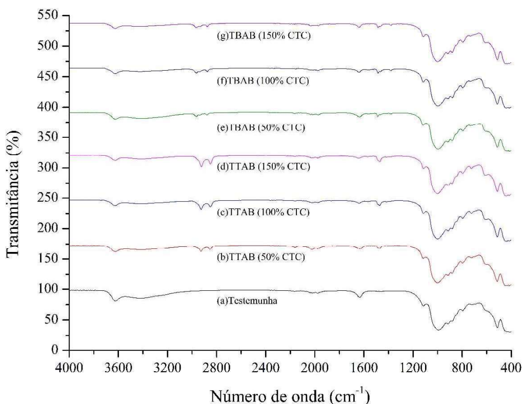
Figura 22. Espectros na região infravermelho da nanoargila não tratada e das nanoargilas organofilizadas.
