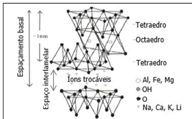
Figura 3. Representação esquemática da estrutura de camadas da montmorilonita. Fonte: Adaptado de FENG et al. (2017).
