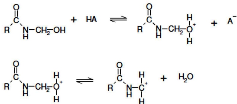
Figura 12. Formação de novos carbocátions. Fonte: LESSMANN (2008).
