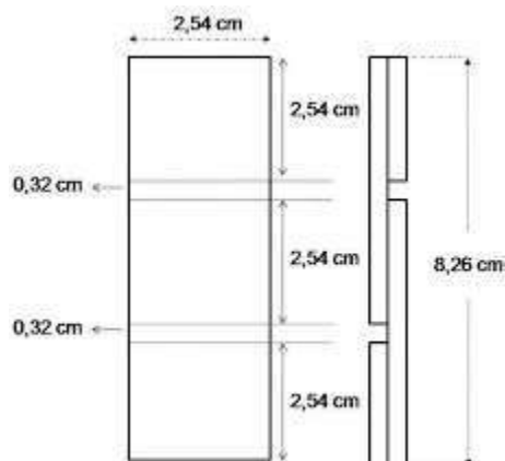
Figura 17. Representação esquemática do corpo de prova utilizado para determinação da resistência ao cisalhamento. Fonte: Adaptado de ASTM (2017).
