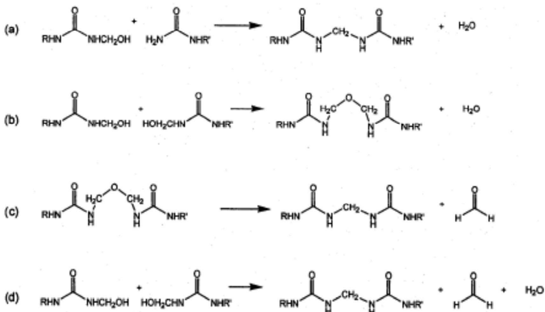
Figura 14. Reações de condensação das metilolureias. Fonte: CONNER (2001).
