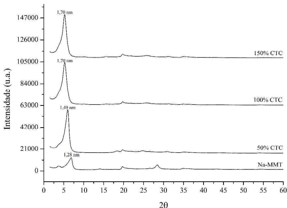
Figura 21. Difratogramas das nanoargilas modificadas com o TBAB.
