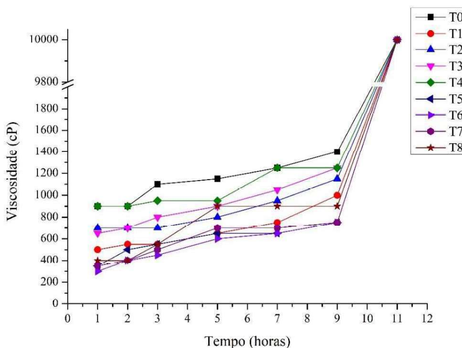
Figura 26. Tempo de trabalho dos adesivos em função dos tratamentos.
