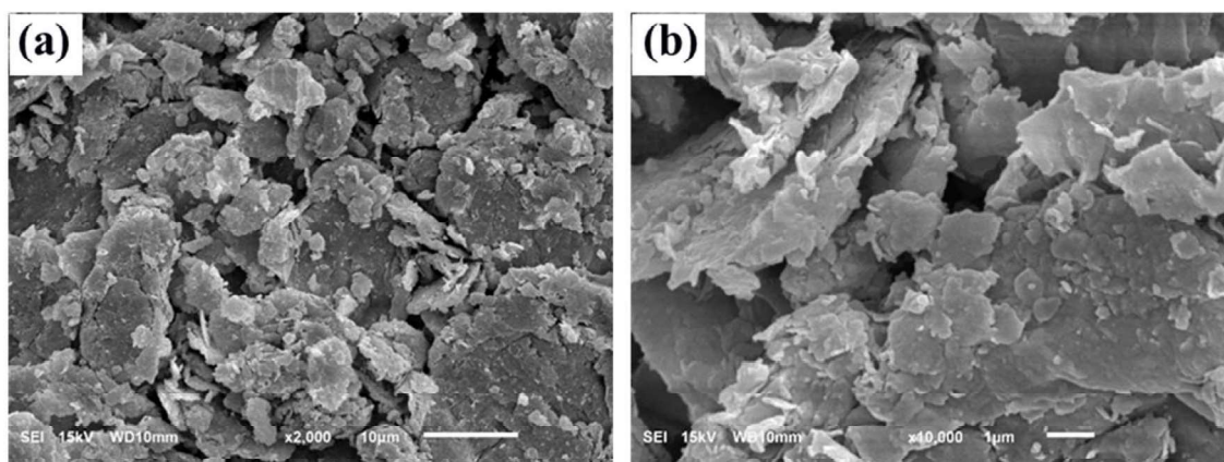
Figura 23. Micrografias obtidas por MEV das nanoargilas (a) não tratada com aumento de 2000x e (b) não tratada com aumento de 10000x.
