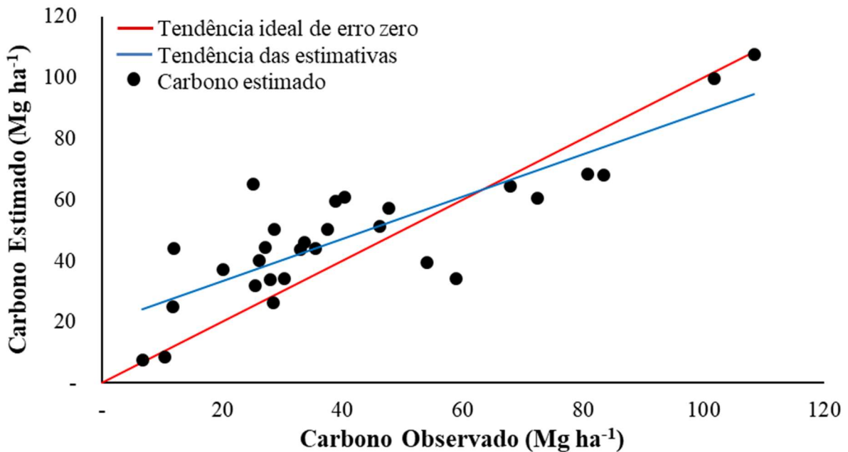
Figura 12 – Média do estoque de carbono por parcela estimado pela RNA treinada com as reflectâncias do período chuvoso, em função do estoque observado nos diferentes estratos sucessionais dos fragmentos florestais da UFV Viçosa.
