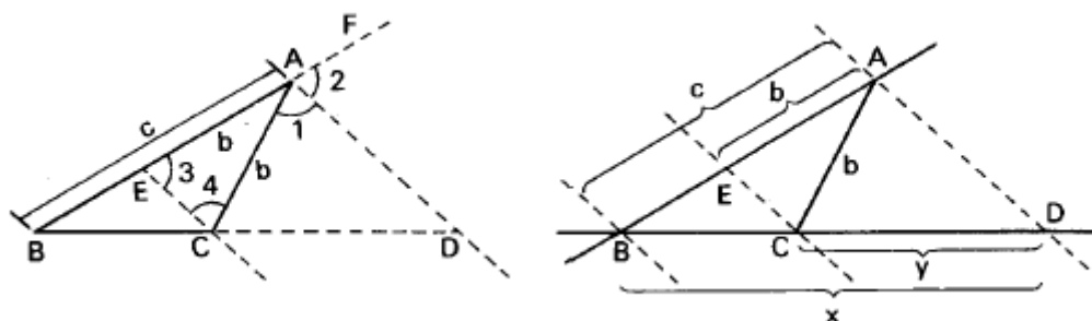
Figura 4.11: Bissetrizes-4, [29].
