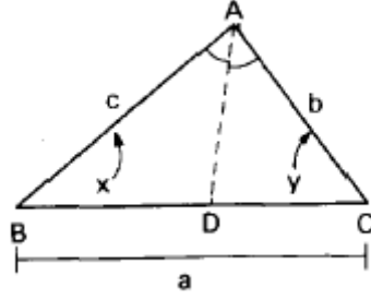
Figura 4.8: Bissetrizes-1, [29].
