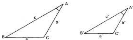
Figura 4.21: Semelhança-5, [29].
