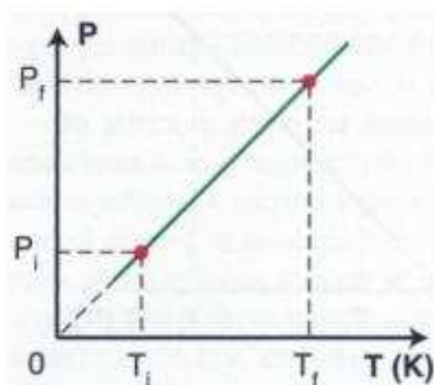
Figura 8.26: http://www.ebah.com.br/content/ABAAAAPp8AF/estudo-fisico-dos-gases?part=2
