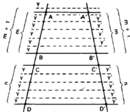
Figura 4.7: Tales-5, [29].
