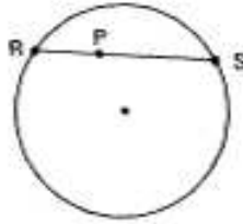
Figura 4.23: Potência-1, [29].
