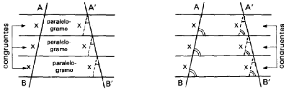
Figura 4.5: Tales-3, [29].
