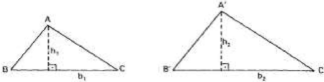
Figura 4.33: Áreas semelhantes-1, [29].
