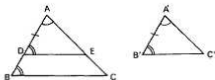
Figura 4.20: Semelhança-4, [29].
