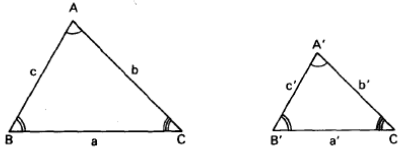
Figura 4.13: Semelhança-1, [29].
