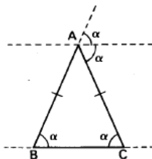
Figura 4.12: Bissetrizes-5, [29].
