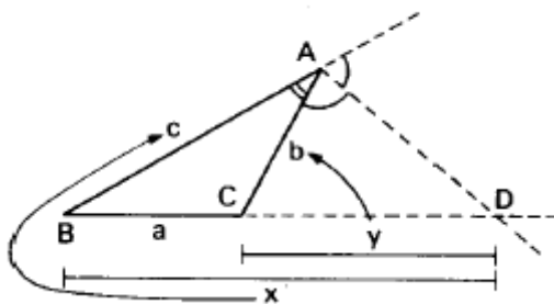
Figura 4.10: Bissetrizes-3, [29].
