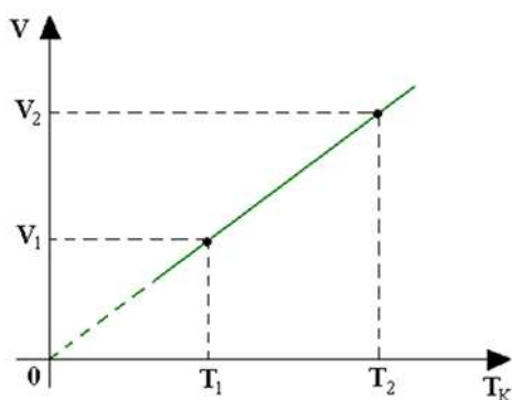
Figura 8.25: http://pt.wikipedia.org/wiki/Transforma%C3%A7%C3%A3o_isob%C3%A1rica
