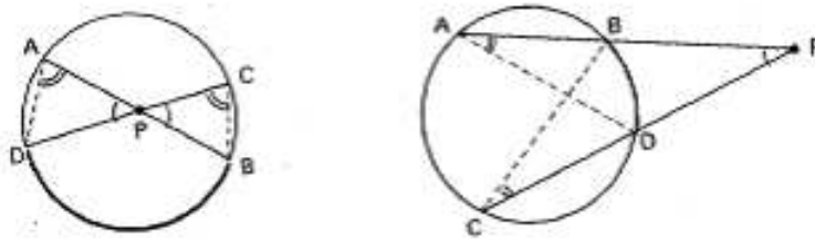
Figura 4.25: Potência-3, [29].
