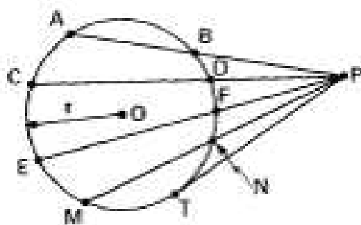
Figura 4.28: Potência-6, [29].
