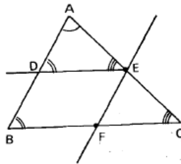
Figura 4.15: Semelhança-3, [29].
