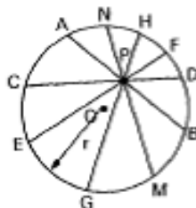
Figura 4.26: Potência-4, [29].
