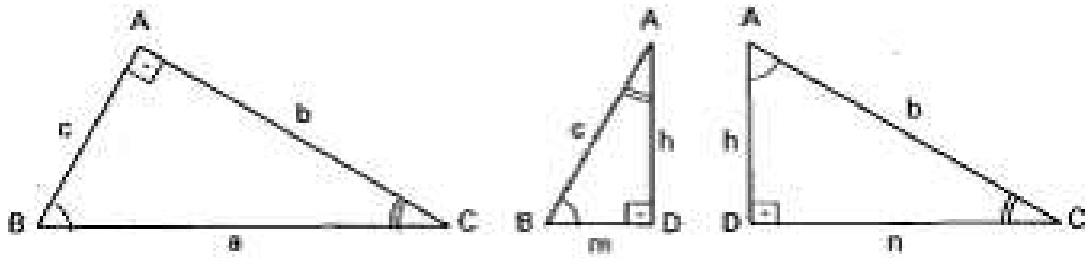
Figura 4.32: Triângulo Retângulo-4, [29].
