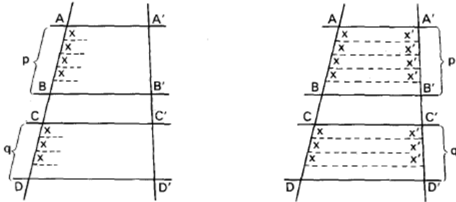
Figura 4.6: Tales-4, [29].
