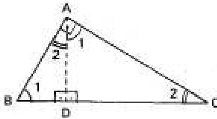
Figura 4.30: Triângulo Retângulo-2, [29].
