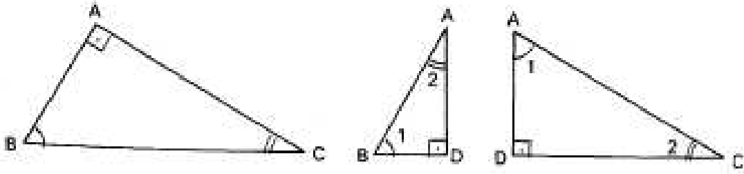
Figura 4.31: Triângulo Retângulo-3, [29].
