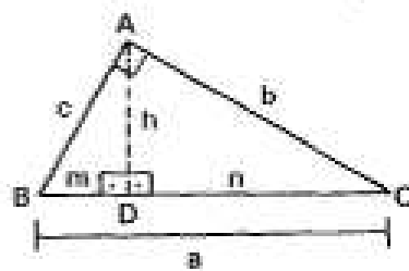
Figura 4.29: Triângulo Retângulo-1, [29].
