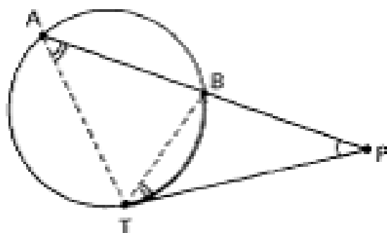
Figura 4.27: Potência-5, [29].
