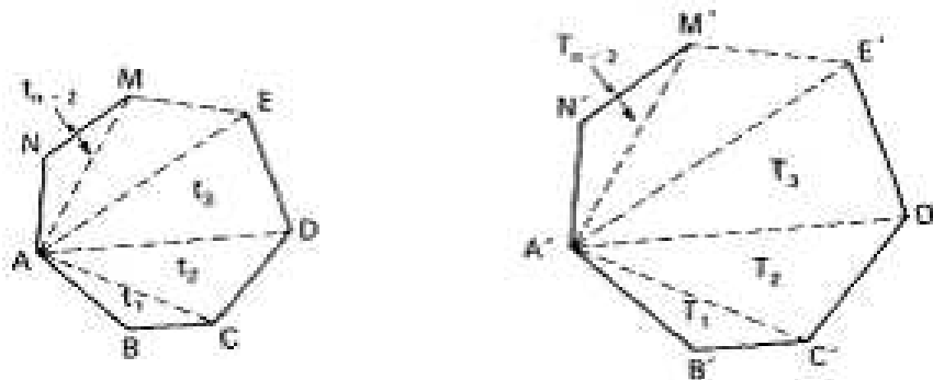
Figura 4.34: Áreas semelhantes-2, [29].
