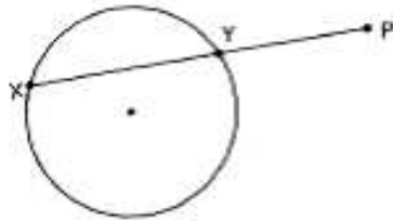
Figura 4.24: Potência-2, [29].
