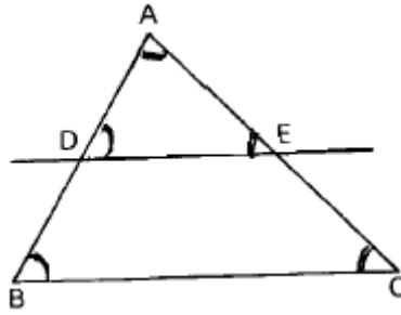
Figura 4.14: Semelhança-2, [29].
