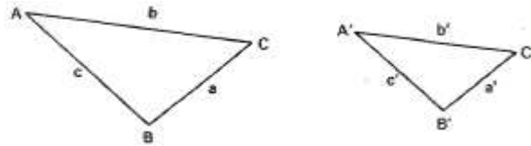
Figura 4.22: Semelhança-6, [29].
