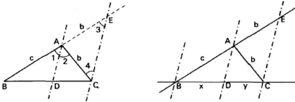
Figura 4.9: Bissetrizes-2, [29].
