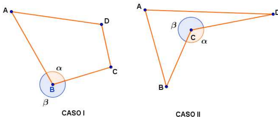
Figura 5.6: Ângulo suplementar.
