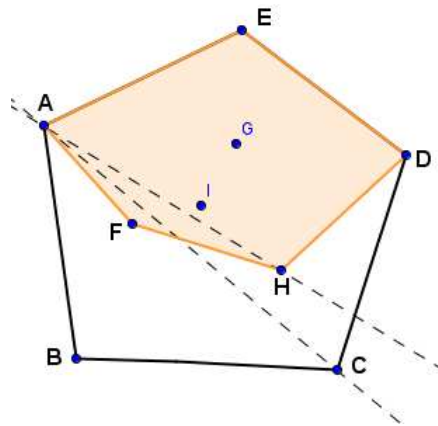
Figura 6.13: Pentágono AEDHF
