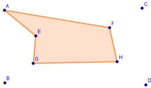
Figura 6.32: Pentágono AFHGE .
