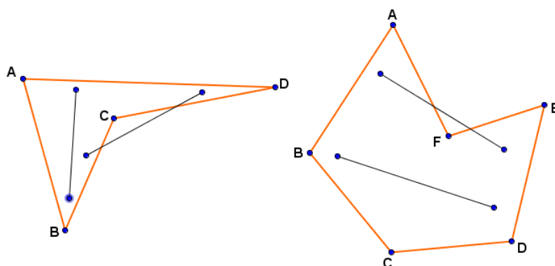
Figura 5.5: Polígonos não-convexos.
