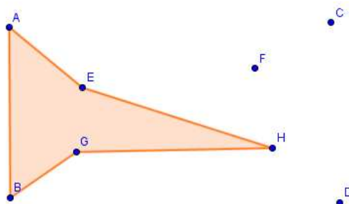
Figura 6.33: Pentágono AEHGB .
