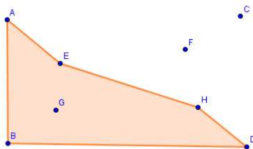
Figura 6.34: Pentágono ABDHE .
