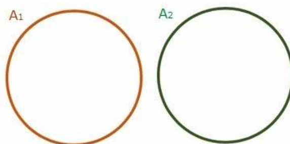
Figura 3.1: Conjuntos disjuntos
