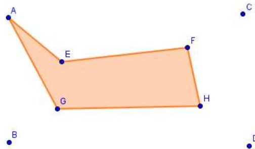
Figura 6.24: Pentágono AGHFE.
