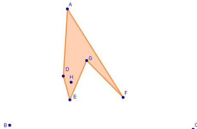
Figura 6.21: Pentágono ADEGF.
