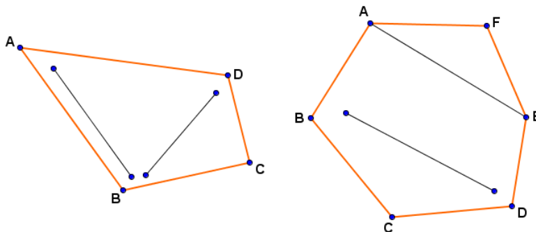
Figura 5.4: Polígonos convexos.
