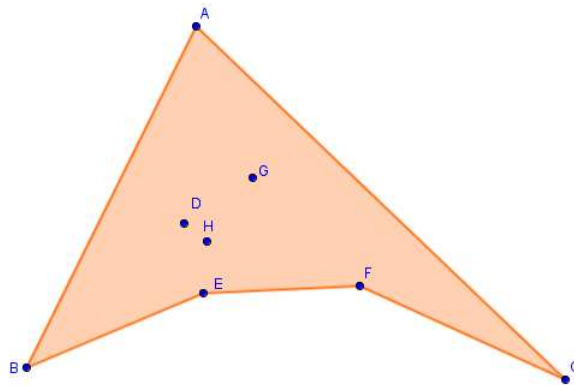
Figura 6.29: Pentágono ABEFC .
