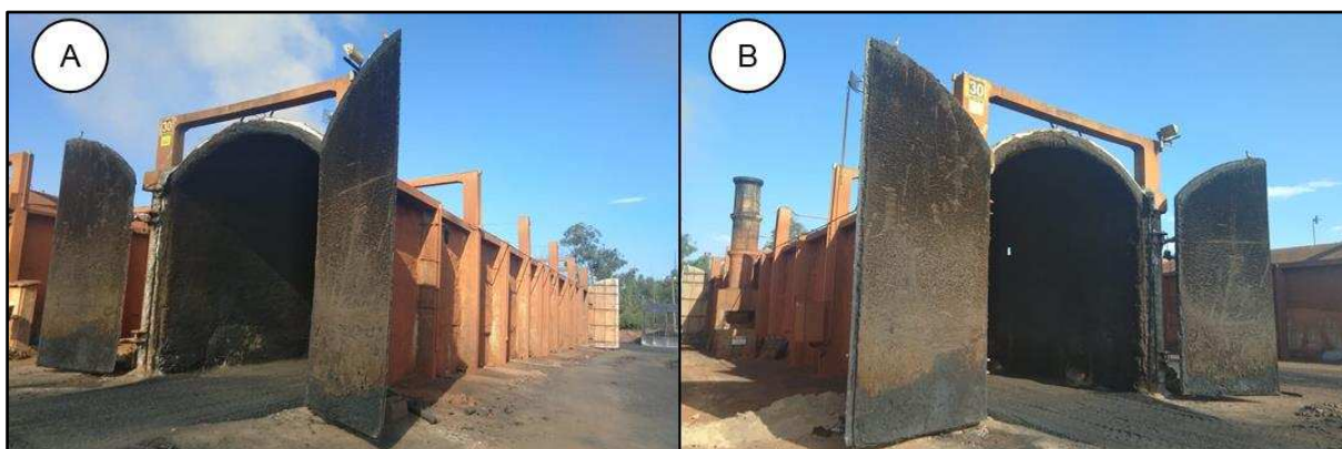
Figura 8 – Forno utilizado para as carbonizações. Vista da parede do lado direito (A) e do lado esquerdo (B) do forno.
