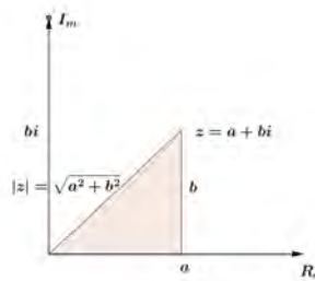
Figura 6.0.2: Representação geométrica da definição do módulo de um número complexo .
