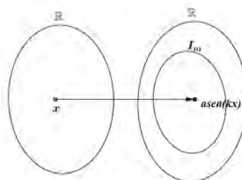
Figura 2.1.1: Diagrama ilustrando a função f(x) = asen(kx) .
