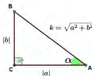
Figura 3.3.1: Triângulo retângulo ABC. \overline{AC} = |a| e \overline{BC} = |b|
