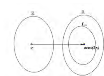
Figura 2.1.2: Diagrama ilustrando a função f(x) = a \cos(kx) .
