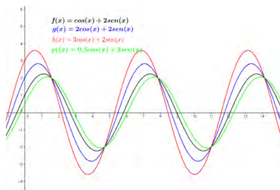
Figura 3.1.2: Gráficos comparativos de alguns monômios trigonométricos da forma p(x) = \alpha \cos(x) + 2 \sin(x) .
