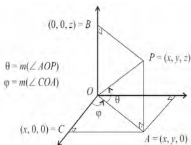
Figura 7.2.1: Coordenadas cartesianas do ponto P localizado no espaço.
