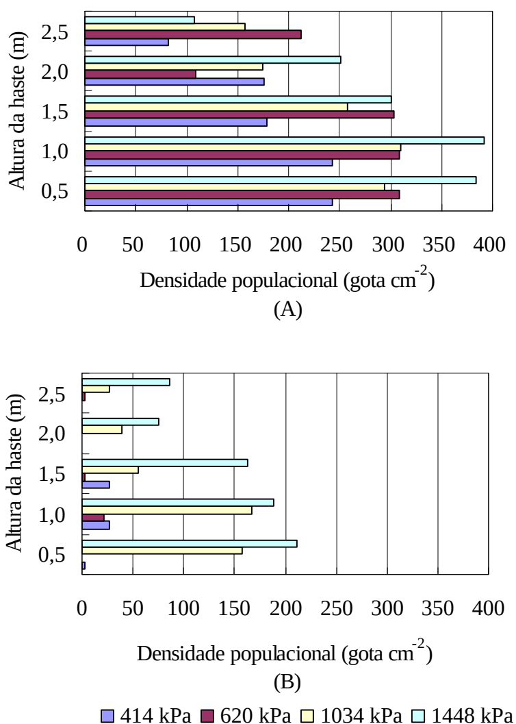
Figura 15. Influência das pressões de trabalho na densidade populacional das gotas proporcionada pelos bicos hidráulicos JA-1, nas rotações do ventilador de 1.860 (A) e 2.160 rpm (B) e velocidade do trator de 6,35 km h -1 .
