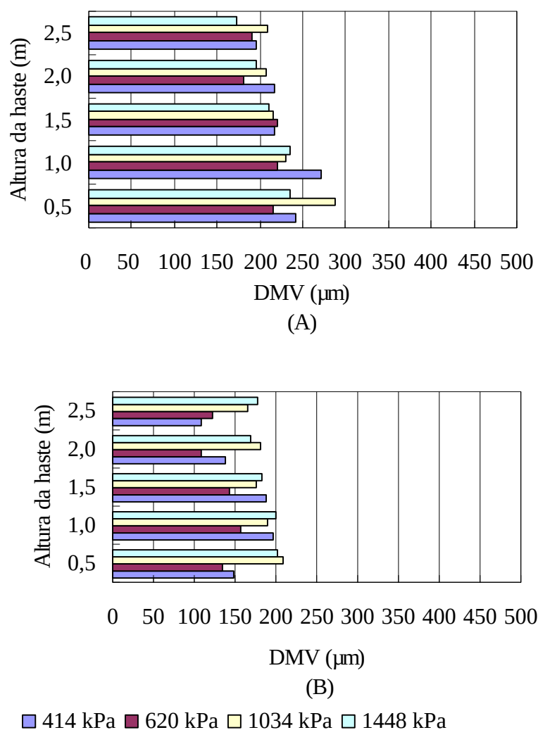
Figura 17. Influência das pressões de trabalho no diâmetro da mediana volumétrica (DMV) proporcionada pelos bicos hidráulicos JA-1, nas rotações do ventilador de 1.860 (A) e 2.160 rpm (B) e velocidade do trator de 6,35 km h -1 .
