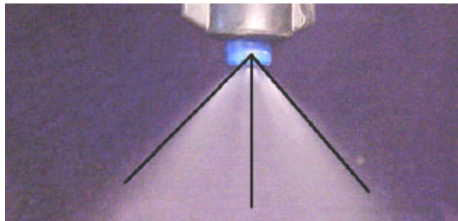
Figura 2. Modelo de imagem utilizada para determinação do ângulo de abertura do jato de pulverização propiciado pelos bicos.
