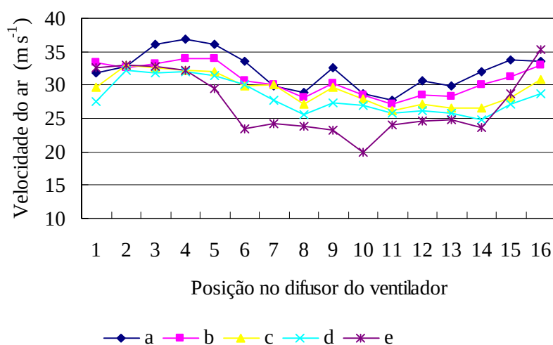
Figura 9. Velocidade do ar na saída do ventilador nas seções a, b, c, d e e, com a velocidade do rotor de 1.960 rpm.
