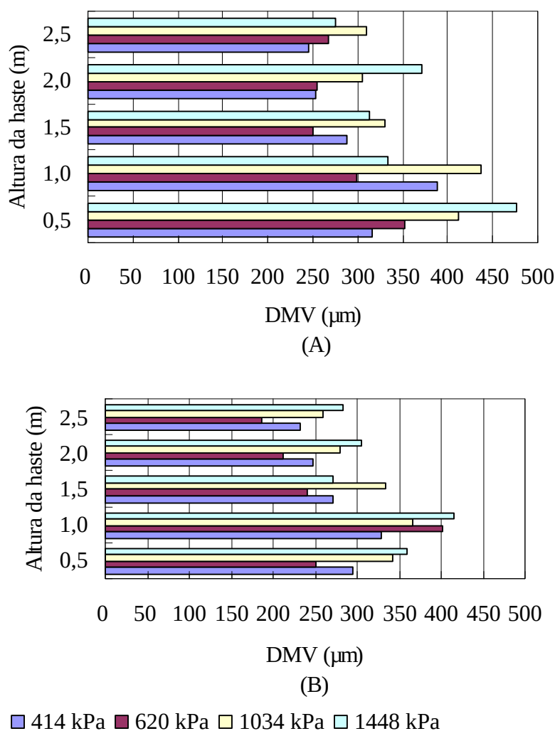
Figura 18. Influência das pressões de trabalho no diâmetro da mediana volumétrica proporcionada pelos bicos hidráulicos JA-2, nas rotações do ventilador de 1.860 (A) e 2.160 rpm (B) e velocidade do trator de 6,35 km h -1 .
