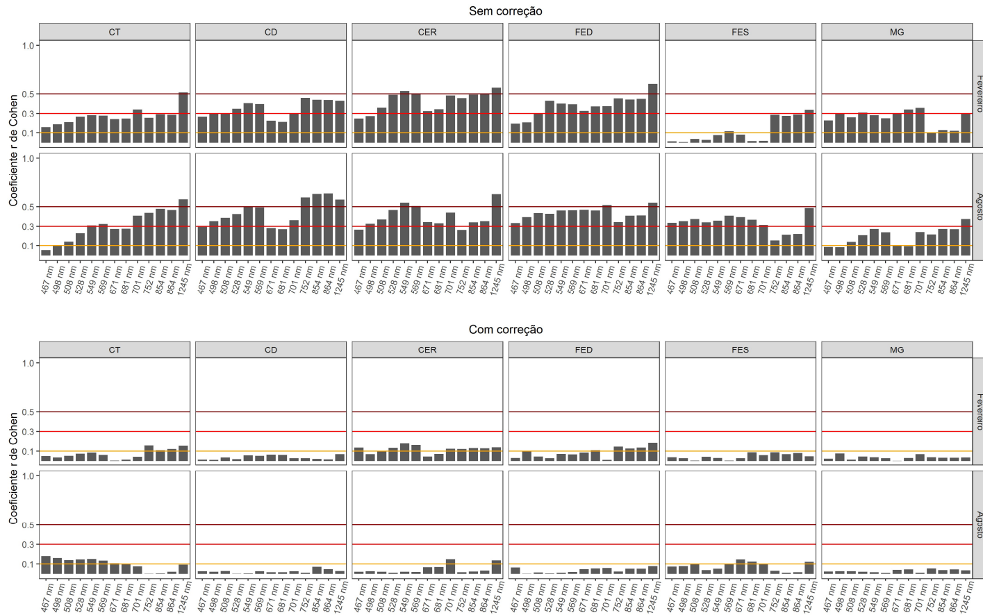
Figura 6 – Magnitude do efeito da geometria de iluminação sobre os valores reamostrados das bandas para as seis fisionomias durante as estações chuvosa (fevereiro) e seca (agosto), antes e após a correção. Valores abaixo da linha amarela ( < 0,1 ) indicam efeito nulo, entre as linhas amarelo e vermelho ( 0,1 - 0,3 ) efeito pequeno, entre as linhas vermelho e vermelho escuro ( 0,3 - 0,5 ) efeito moderado e acima da linha vermelho escuro ( > 0,5 ) efeito grande. CT = Cerrado Típico, CD = Cerrado Denso, CER = Cerradão, FED = Floresta Estacional Decidual, FES = Floresta Estacional Semidecidual, MG = Mata de Galeria.
