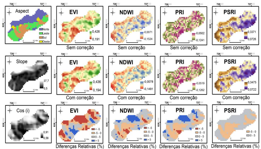
Figura 10 – Índices EVI, NDWI, PRI e PSRI corrigidos e não-corrigidos, e suas respectivas diferenças relativas em porcentagem para um fragmento de Cerrado Denso durante as estações chuvosa (fevereiro) e seca (agosto).
