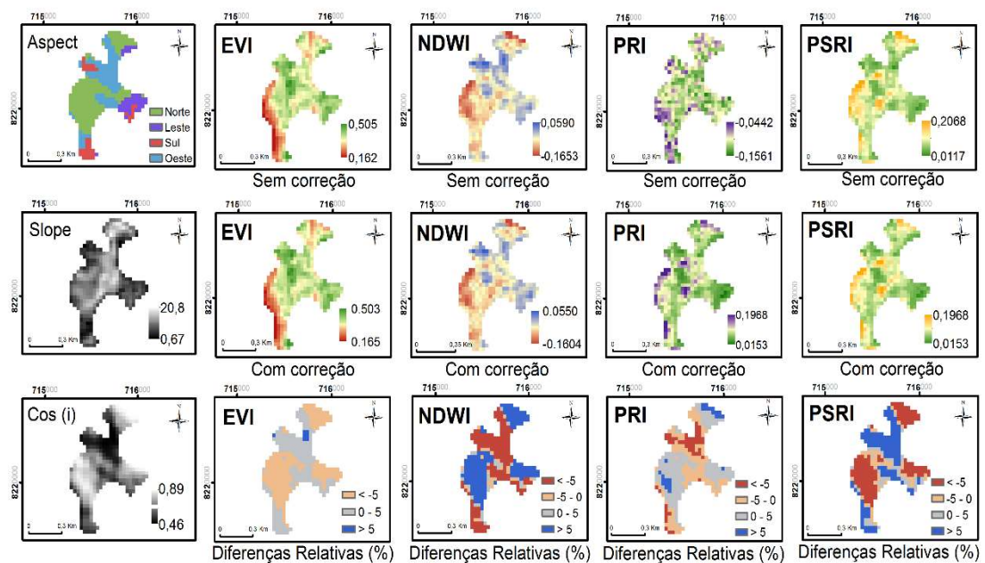
Figura 11 – Índices EVI, NDWI, PRI e PSRI corrigidos e não-corrigidos, e suas respectivas diferenças relativas em porcentagem para um fragmento de Floresta Estacional Semidecidual durante as estações chuvosa (fevereiro) e seca (agosto).
