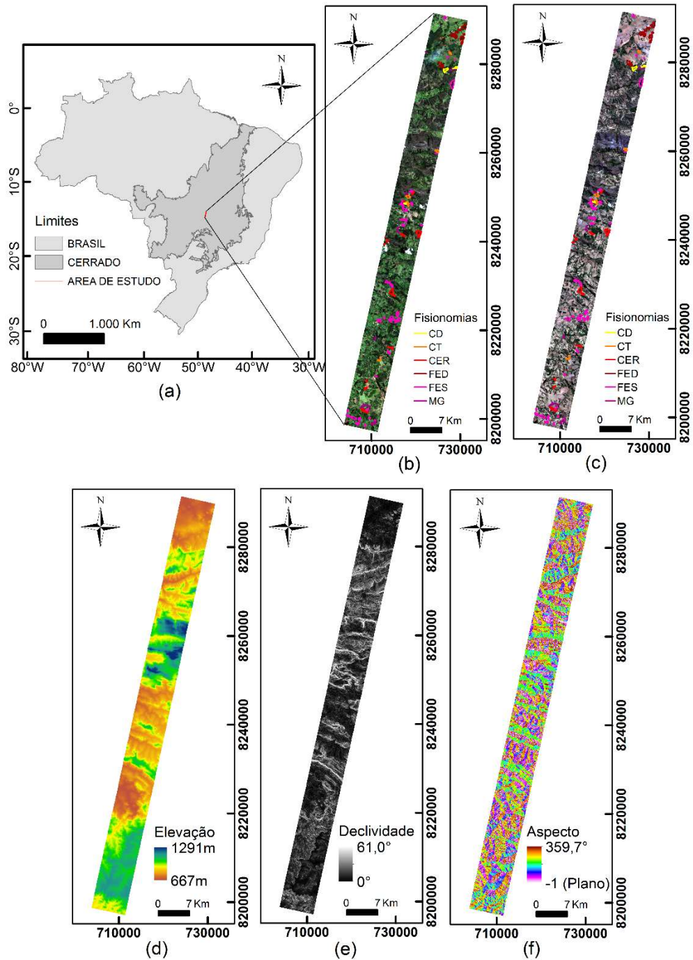
Figura 1 - Área de estudo. (a) – Localização da área no Cerrado brasileiro; (b) – Composição em cores reais da área durante a estação chuvosa (fevereiro), CT = Cerrado Típico, CD = Cerrado Denso, CER = Cerradão, FED = Floresta Estacional Decidual, FES = Floresta Estacional Semidecidual, MG = Mata de Galeria; (c) – Composição em cores reais da área durante a estação seca (agosto), CT = Cerrado Típico, CD = Cerrado Denso, CER = Cerradão, FED = Floresta Estacional Decidual, FES = Floresta Estacional Semidecidual, MG = Mata de Galeria; (d) – Modelo digital de elevação da área (metros); (e) – Declividade da área (graus); (f) – Aspecto (faces de exposição do terreno) da área (graus).
