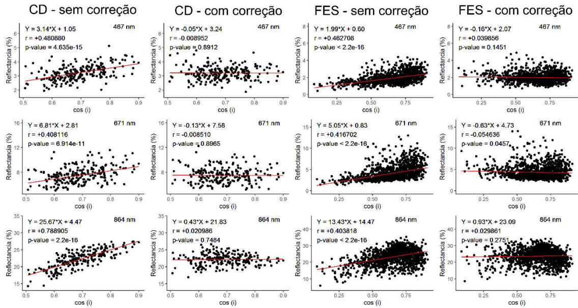
Figura 2 – Gráficos das regressões entre o cos (i) e a reflectância das bandas 12 (467 nm), 32 (671 nm) e 51 (864 nm) antes e após a correção topográfica, para as fisionomias Cerrado Denso (CD) e Floresta Estacional Semidecidual (FES) em agosto.
