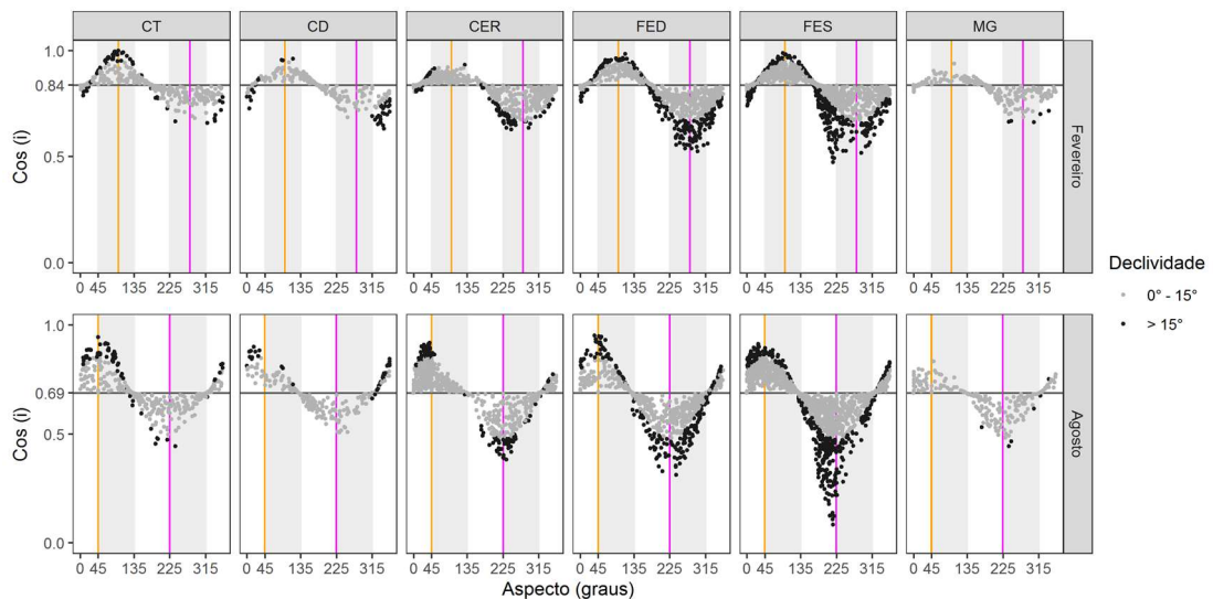
Figura 5 – Distribuição dos valores do \cos(i) ao longo das faces de exposição (aspecto) para as fisionomias nas duas datas. As diferentes cores dos pontos indicam onde a declividade é maior ou menor que quinze graus. As linhas horizontais que separam as classes sombreada e iluminada representam onde \cos(i) = \cos(\theta_z) em cada data. As linhas coloridas verticais representam os valores dos ângulos de azimute solar ( \phi_s ) (laranja) e da face oposta ao azimute ( \phi_s + 180^\circ ) (magenta) em cada data.
