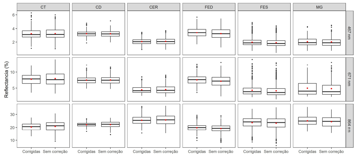
Figura 3 – boxplots com os valores das reflectâncias (%) para as bandas 12 (azul), 32
