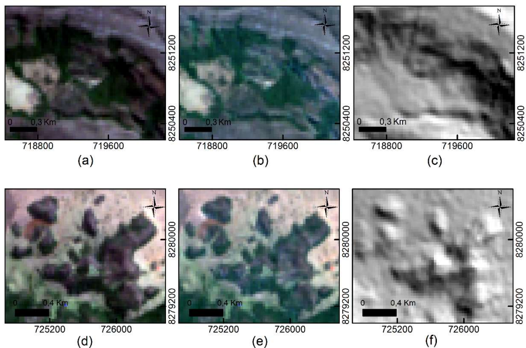
Figura 4 – Efeito da iluminação do terreno e da correção topográfica sobre a reflectância em algumas fitosifionomias. (a) – Composição RGB de um fragmento de Floresta Estacional Semidecidual em agosto antes da correção; (b) – Composição RGB após a correção; (c) – imagem do cos (i) para a área em questão; (d) – Composição RGB de um fragmento de Floresta Estacional Decidual em agosto antes da correção; (e) – Composição RGB após a correção; (f) – imagem do cos (i) para a área em questão;
