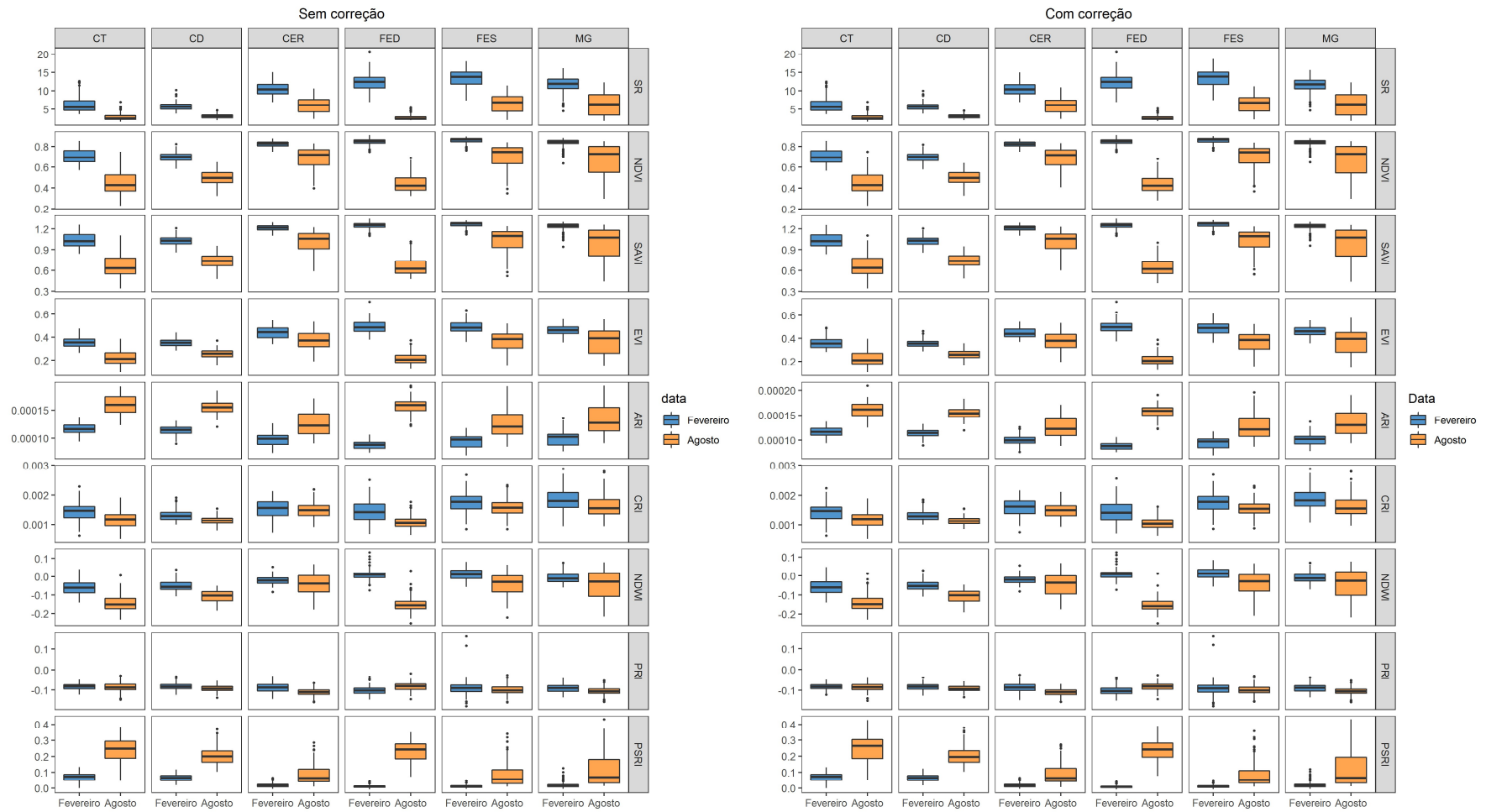
Figura 12 – Boxplot dos valores dos índices hiperespectrais nas estações chuvosa (fevereiro) e seca (agosto), em todas as fisionomias, antes e após a correção topográfica. CT = Cerrado Típico, CD = Cerrado Denso, CER = Cerradão, FED = Floresta Estacional Decidual, FES = Floresta Estacional Semidecidual, MG = Mata de Galeria.
