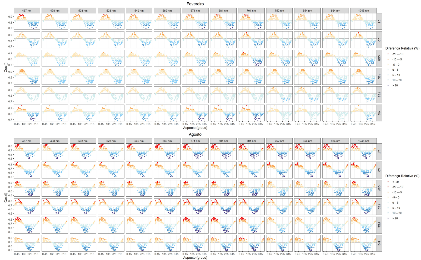
Figura 7 - Distribuição dos valores do \text{Cos}(i) ao longo das faces de exposição (aspecto) para as bandas nas seis fisionomias durante as estações chuvosa (fevereiro) e seca (agosto). As diferentes cores dos pontos representam as amplitudes de diferenças relativas (%) entre os pixels não-corrigidos e corrigidos. CT = Cerrado Típico, CD = Cerrado Denso, CER = Cerradão, FED = Floresta Estacional Decidual, FES = Floresta Estacional Semidecidual, MG = Mata de Galeria.
