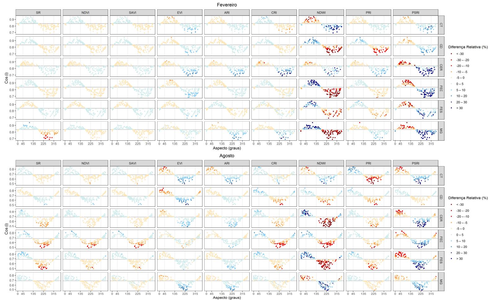
Figura 9 - Distribuição dos valores do \text{Cos}(i) ao longo das faces de exposição (aspecto) para os índices nas seis fisionomias durante as estações chuvosa (fevereiro) e seca (agosto). As diferentes cores dos pontos representam as amplitudes de diferenças relativas (%) entre os pixels não-corrigidos e corrigidos. CT = Cerrado Típico, CD = Cerrado Denso, CER = Cerradão, FED = Floresta Estacional Decidual, FES = Floresta Estacional Semidecidual, MG = Mata de Galeria.
