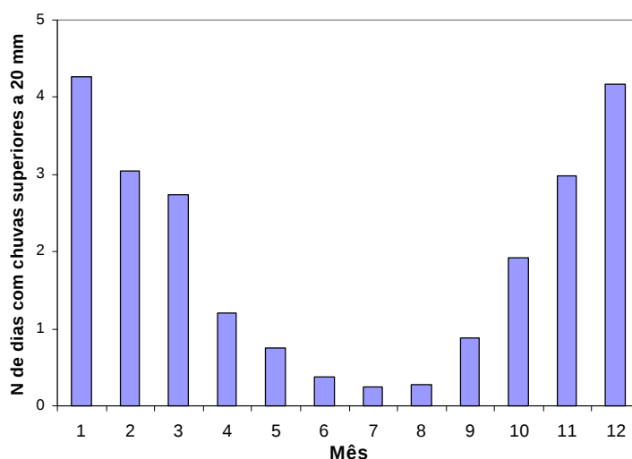
Figura 12. Número de dias com chuvas superiores a 20 mm em cada mês.
