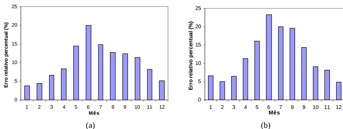
Figura 16. Módulos dos erros relativos percentuais entre a média (a) e o desvio padrão (b) da intensidade de pico na região VI.
