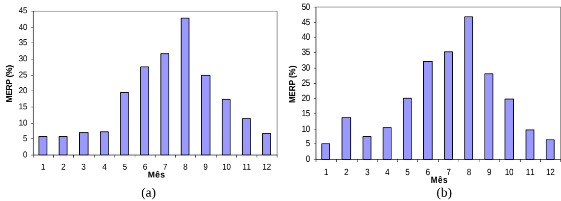
Figura 4F. Módulos dos erros relativos percentuais para a média (a) e o desvio padrão (b) da tempo de pico padronizado na região homogênea IV.
