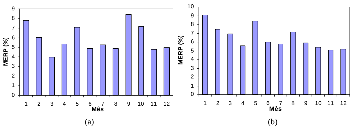
Figura 5D. Módulos dos erros relativos percentuais para a média (a) e o desvio padrão (b) da duração efetiva na região homogênea V.
