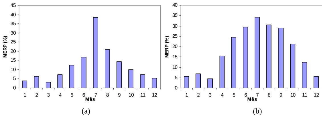
Figura 4D. Módulos dos erros relativos percentuais para a média (a) e o desvio padrão (b) da duração efetiva na região homogênea IV.
