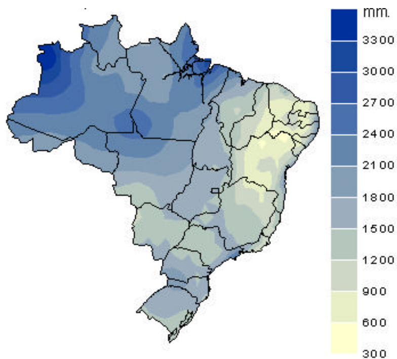
Figura 3. Distribuição da precipitação no Brasil (INMET, 2004).
