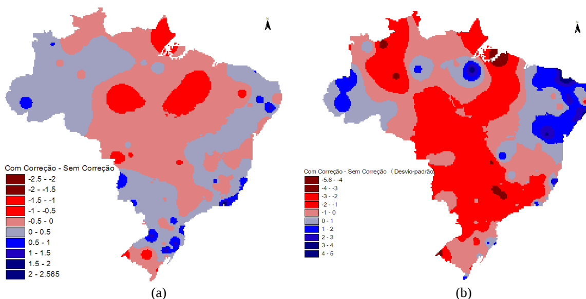
Figura 25. Diferença entre os valores do MERP obtidos com e sem a utilização da correção, para a média (a) e o desvio padrão (b) da temperatura máxima.
