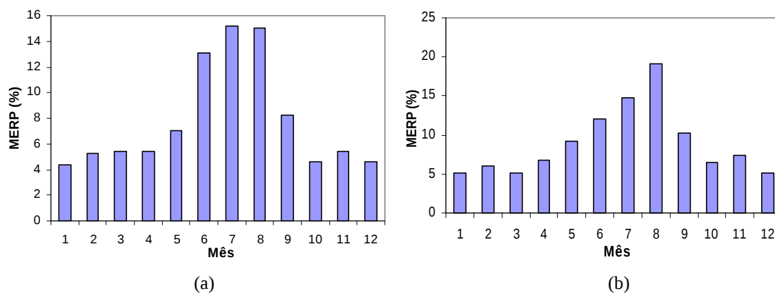
Figura 2E. Módulos dos erros relativos percentuais para a média (a) e o desvio padrão (b) da intensidade de pico na região homogênea II.
