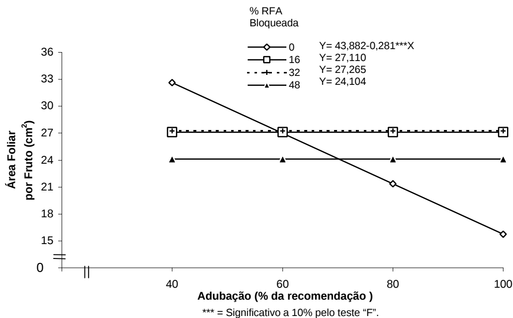
Figura 5. Área foliar por fruto (Y) em função do nível de adubação (X) em cafeeiros submetidos a diferentes níveis de bloqueio de RFA (% Radição fotossinteticamente ativa).
