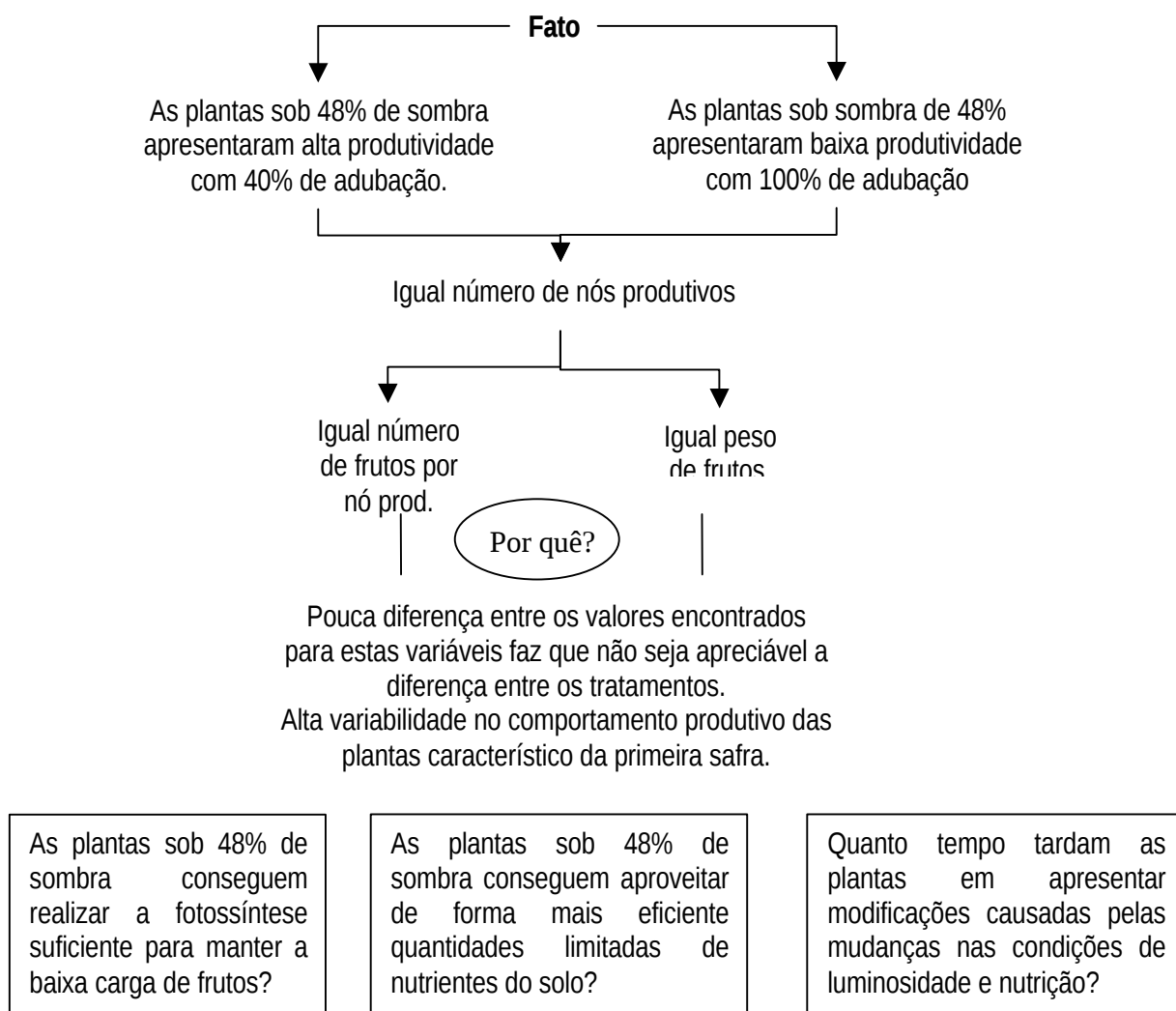
Figura 9. Comportamento das plantas sob 48% de bloqueio da RFA observado durante o experimento, possíveis causas e perguntas que surgem a partir do fato observado.
